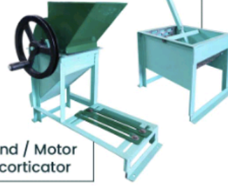
Hand Decorticator
